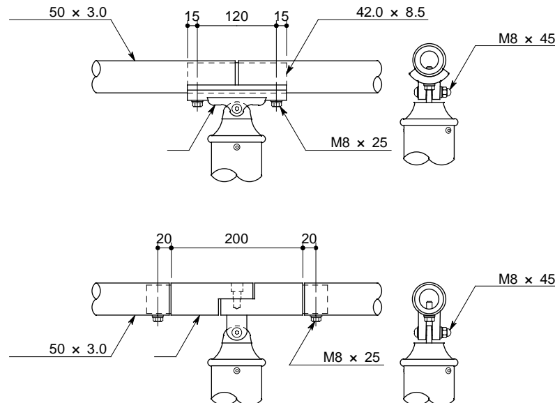
T金具詳細図
