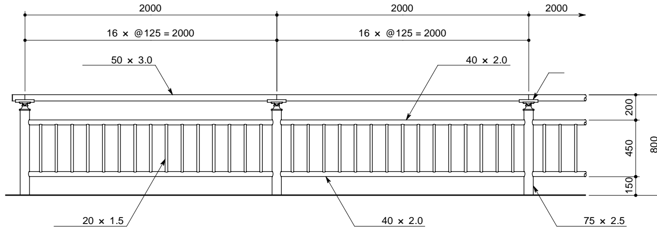
正面図
