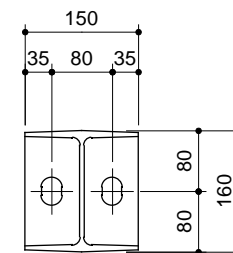
A ~ A断面図
