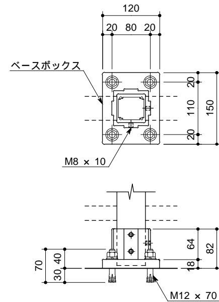
ベース部詳細図
